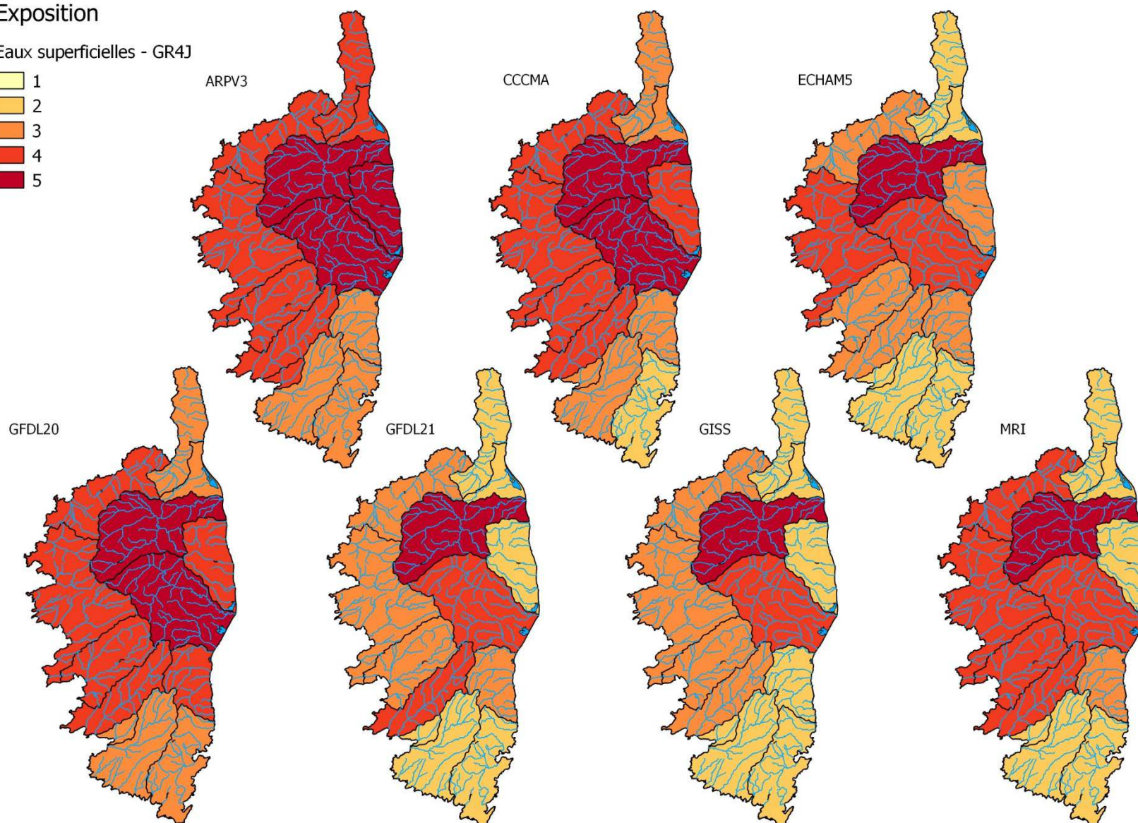
Figure 12 - Exposition des territoires pour l'enjeu disponibilité en eaux superficielles avec les projections GR4J
