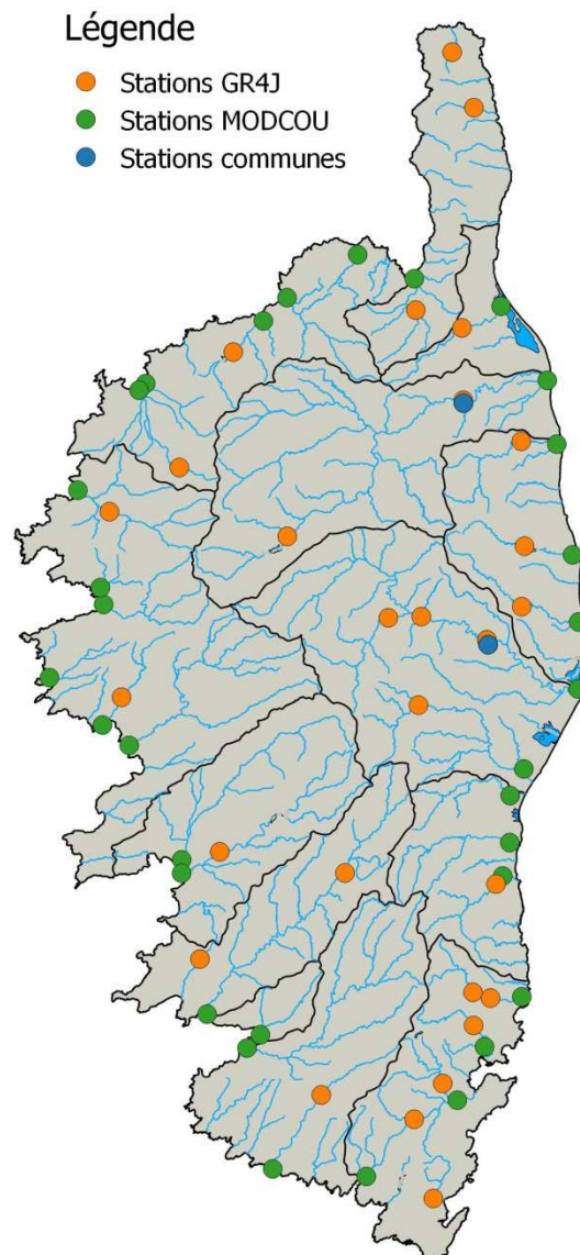
Figure 6 - Points de modélisation disponibles sur le bassin de Corse pour MODCOU et GR4J
